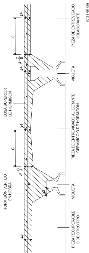
Figura 59.2.1 Condiciones geométricas de los forjados
