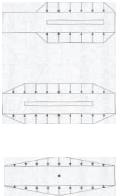
Figura A.12.5.2.4.d. Formas supuestas de las fuerzas cortantes verticales en las juntas
