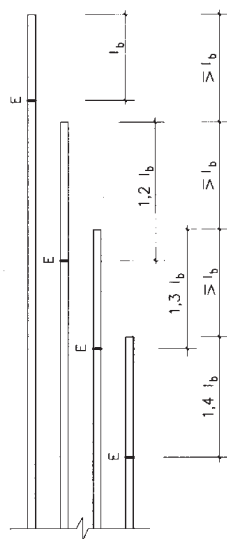
E: SECCIÓN EN QUE DEJA DE SER NECESARIA LA BARRA
