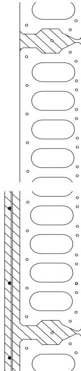
Figura A.12.3.2. Tipos usuales de forjados de losas alveolares prefensadas
