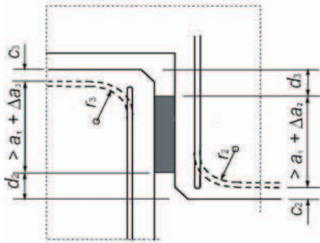
Figura 59.1.3.8.2.b Ejemplo de detalle de armado en un apoyo
