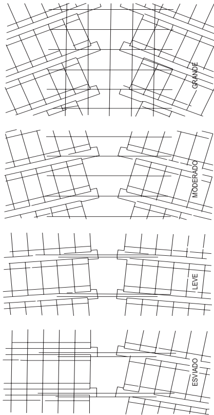
Figura A.12.8.1.c Encuentro oblicuo de viguetas
