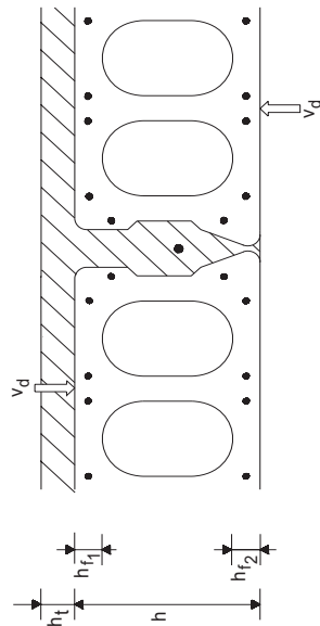
Figura 44.2.3.6 Esfuerzo cortante en las juntas de losas alveolares pretensadas
