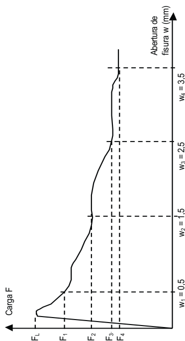
Figura A.14.1. Diagrama tipo carga apertura de fisuras
